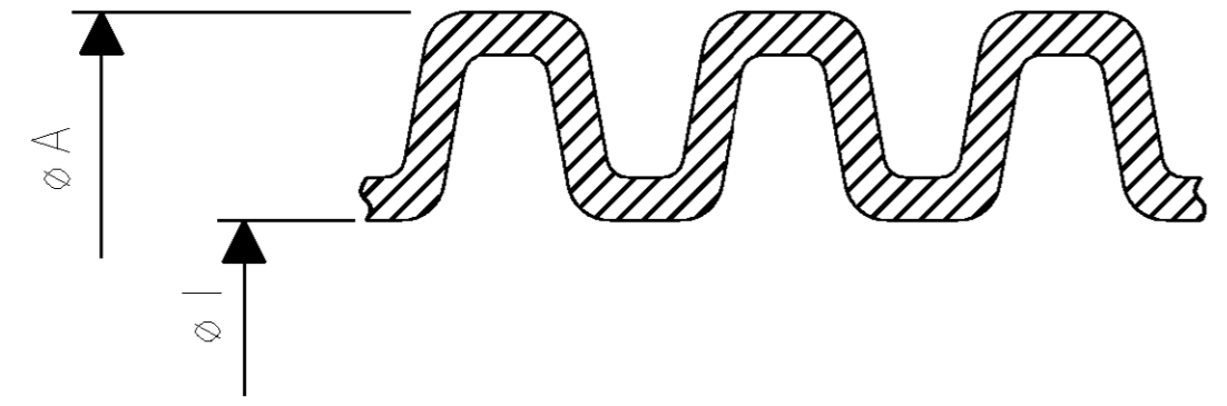
Detail Einzelheit "X"
